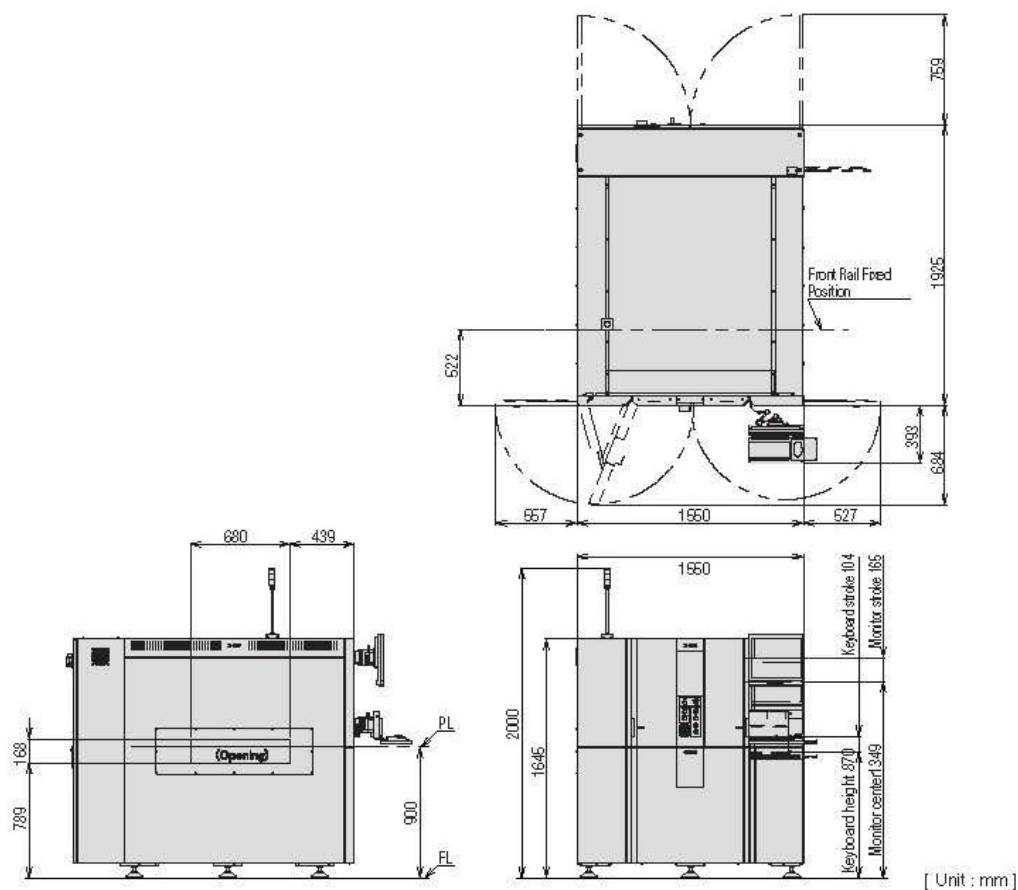
图 9-2 OmronVT-X750 型工业 CT 检测装置外观尺寸图
