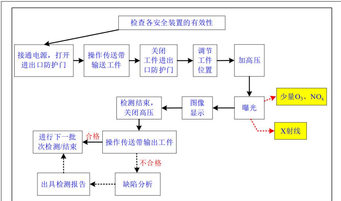
图 9-4 本项目工业 X 射线计算机断层扫描装置工作流程及产污环节示意图
