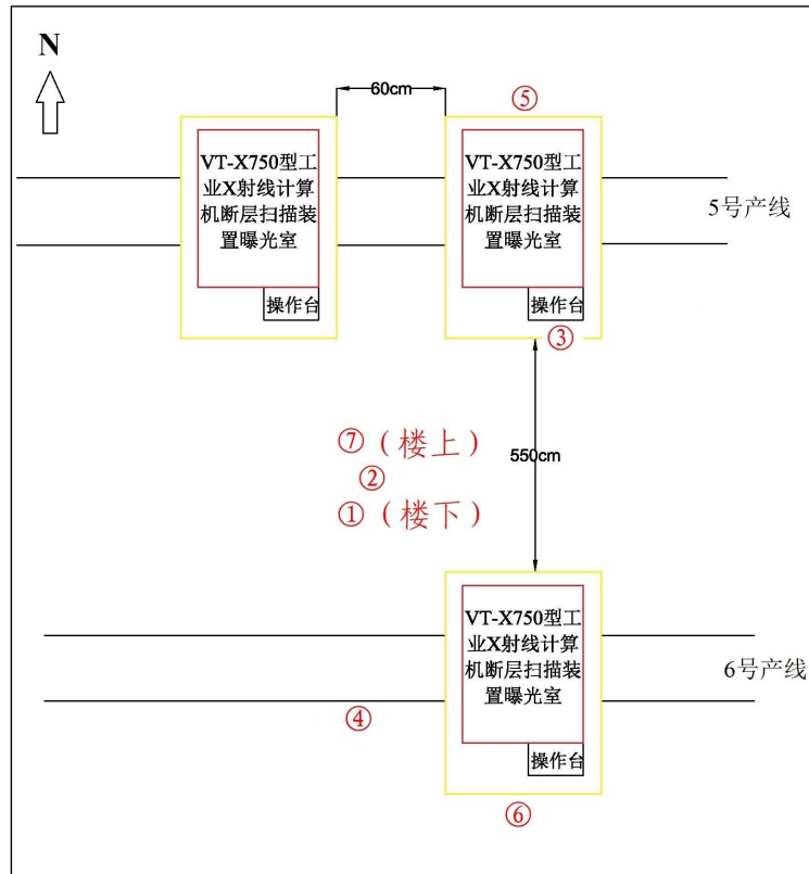
图 11-2 本项目 3 台工业 X 射线计算机断层扫描装置辐射剂量率估算点位示意图
