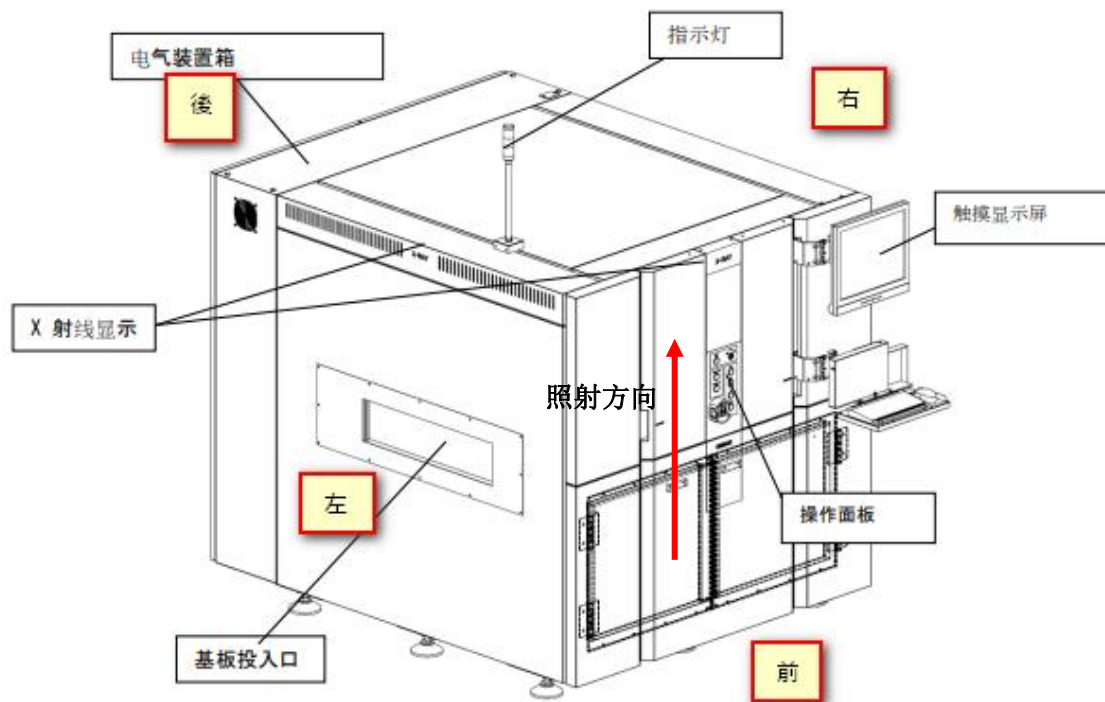
图 9-1 OmronVT-X750 型工业 CT 检测装置样式图
