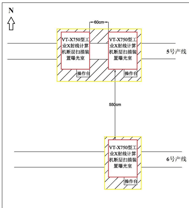
图 10-1 本项目 3 台工业 X 射线计算机断层扫描装置平面布局及分区图
