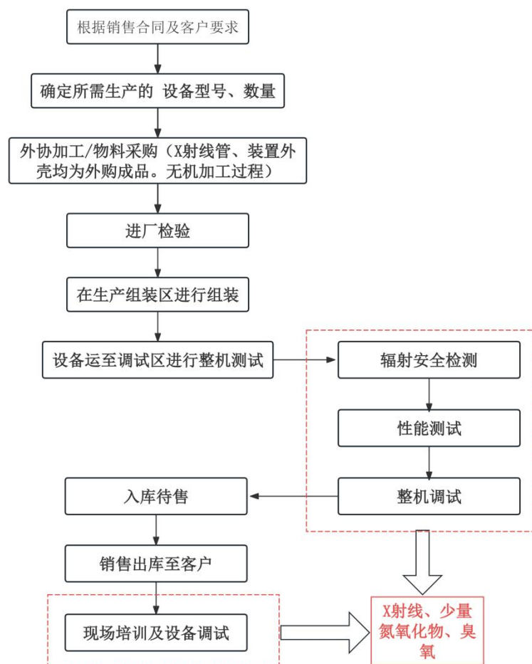
图 9-6 本项目工业 X 射线检测装置的生产、调试、销售流程及产污环节示意图
