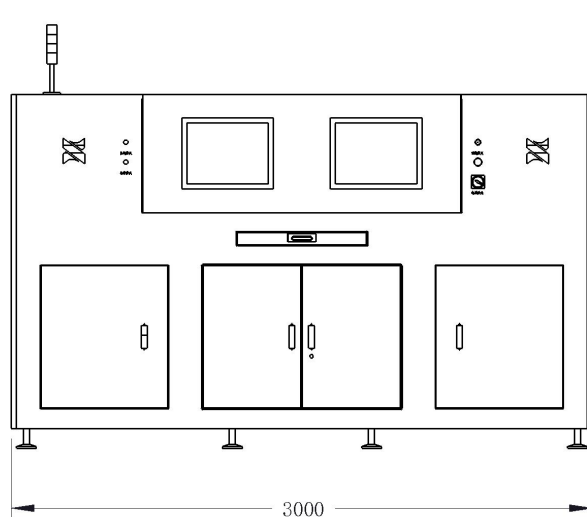
主视图
