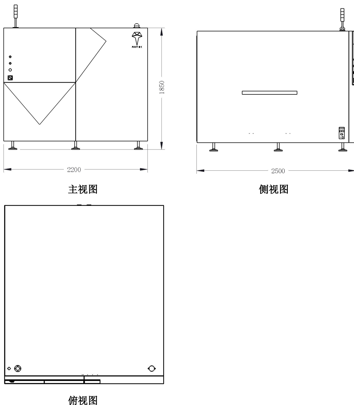
图 9-2 AX1-TD 型工业 X 射线检测装置外观尺寸图（单位：mm）
