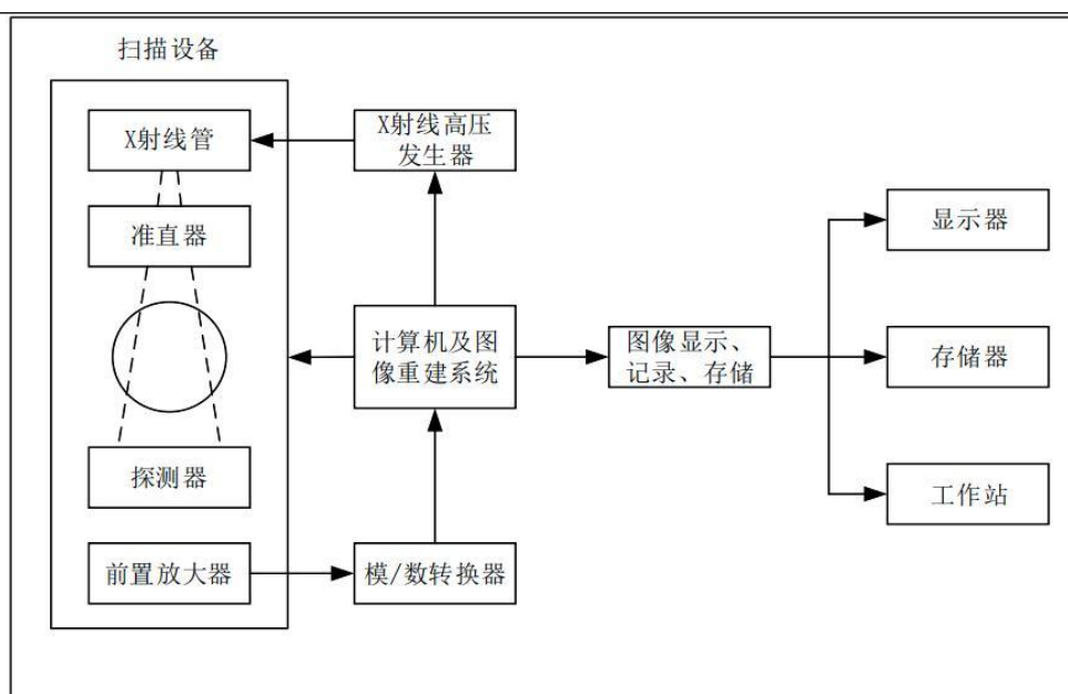
图 9-4 工业 CT 工作原理示意图
