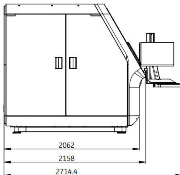
图 9-2 (2) Nanome | x Neo 180X 型 X 射线检测系统侧视图 (单位: mm)
