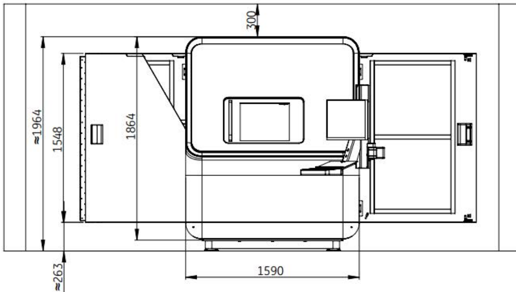
图 9-2 (1) Nanome | x Neo 180X 型 X 射线检测系统正视图 (单位: mm)
