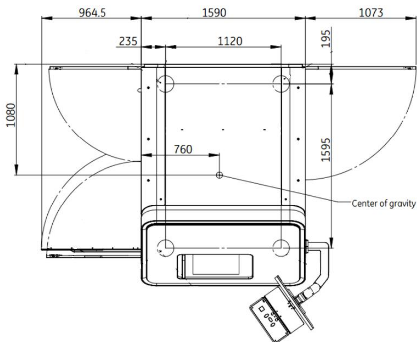
图 9-2（3） Nanome | x Neo 180X 型 X 射线检测系统俯视图（单位：mm）
