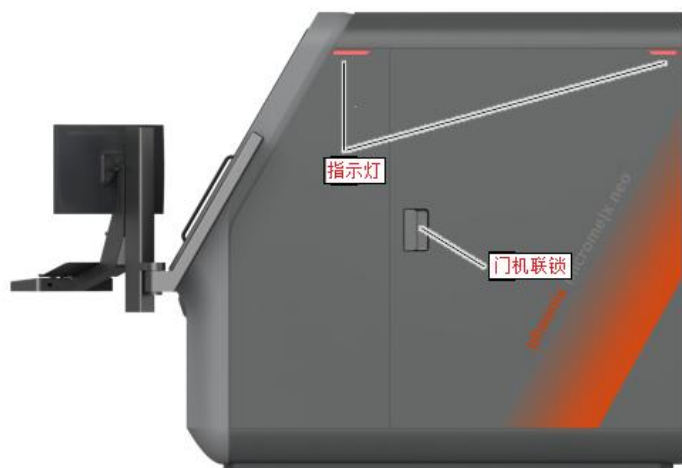
图 10-2 X 射线检测系统辐射安全和防护措施示意图
