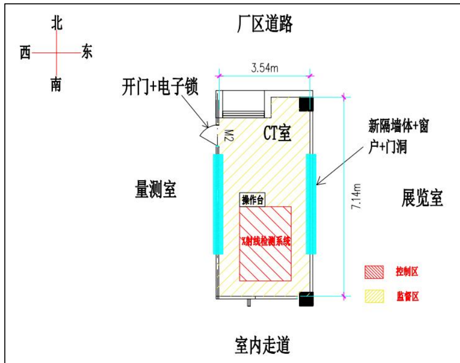
图 10-1 本项目 X 射线检测系统控制分区示意图
