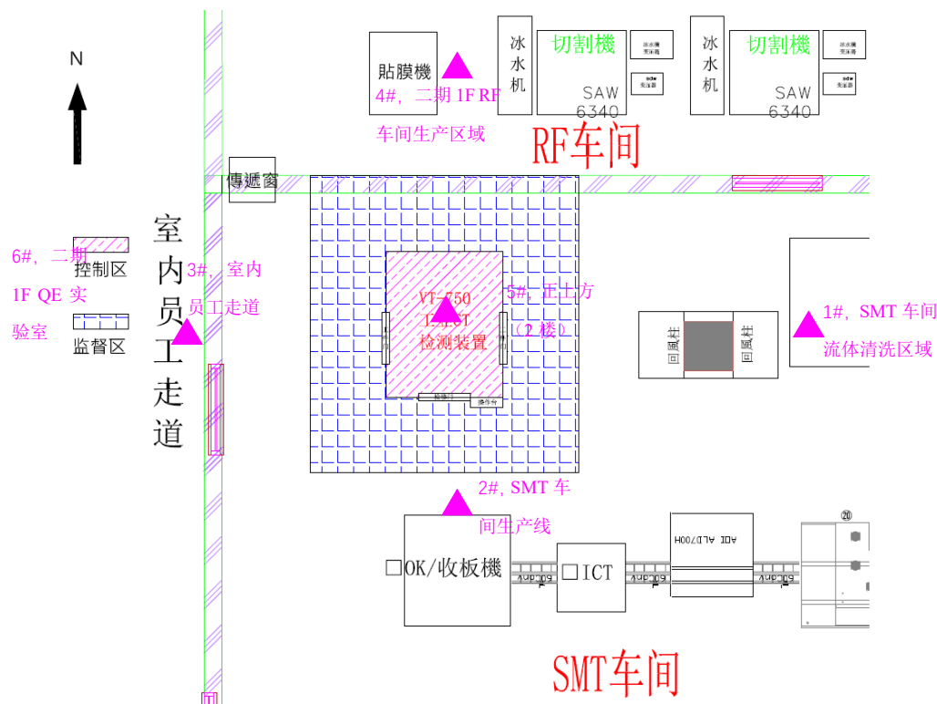
图 11-2 CT 室工业 CT 检测装置周围公众关注点
