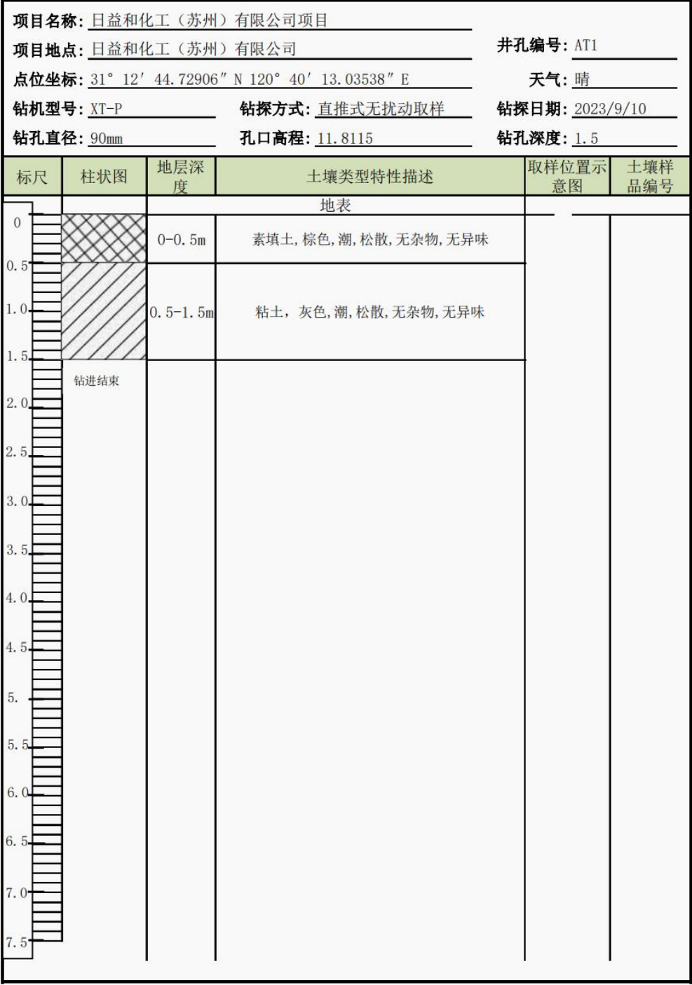
钻孔柱状图
