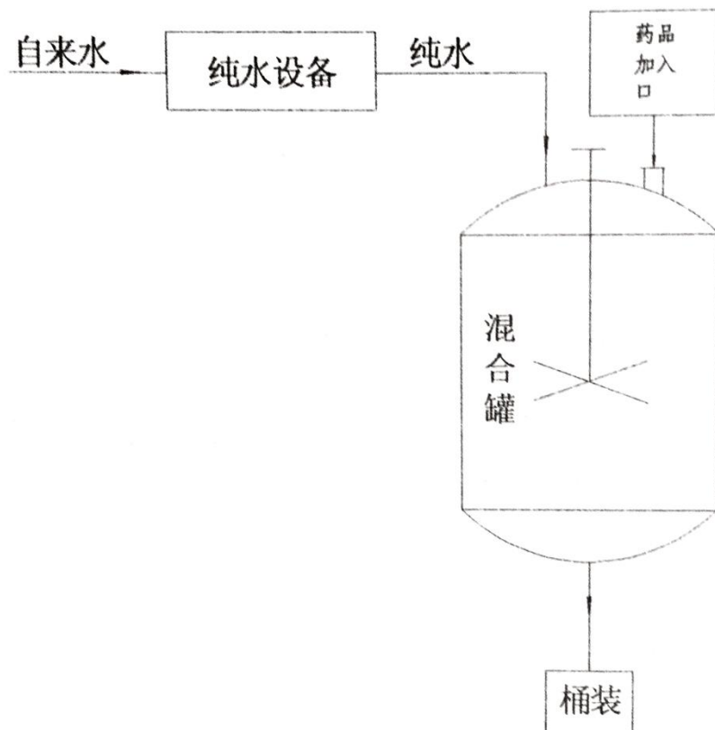
图4.1-1 水处理药剂生产工艺流程图
