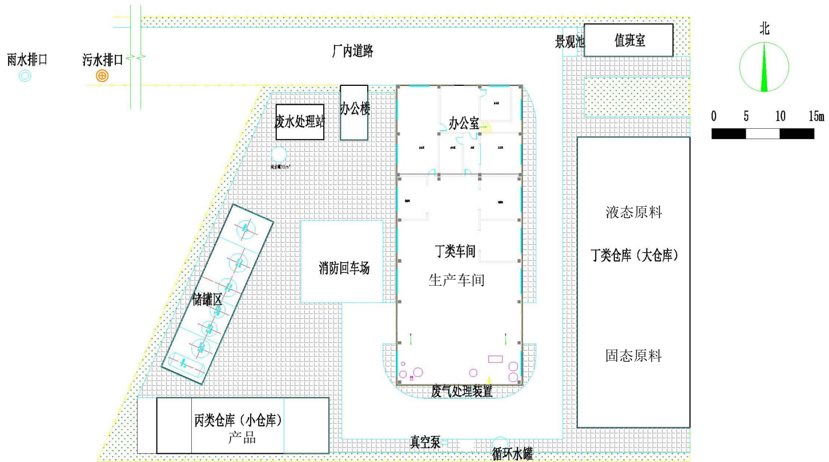
图 4.2-1 项目平面布置图
