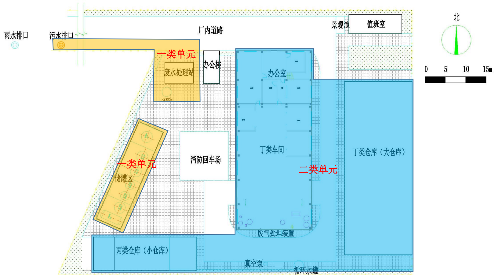
图5.2-1 重点监测单元分区图
