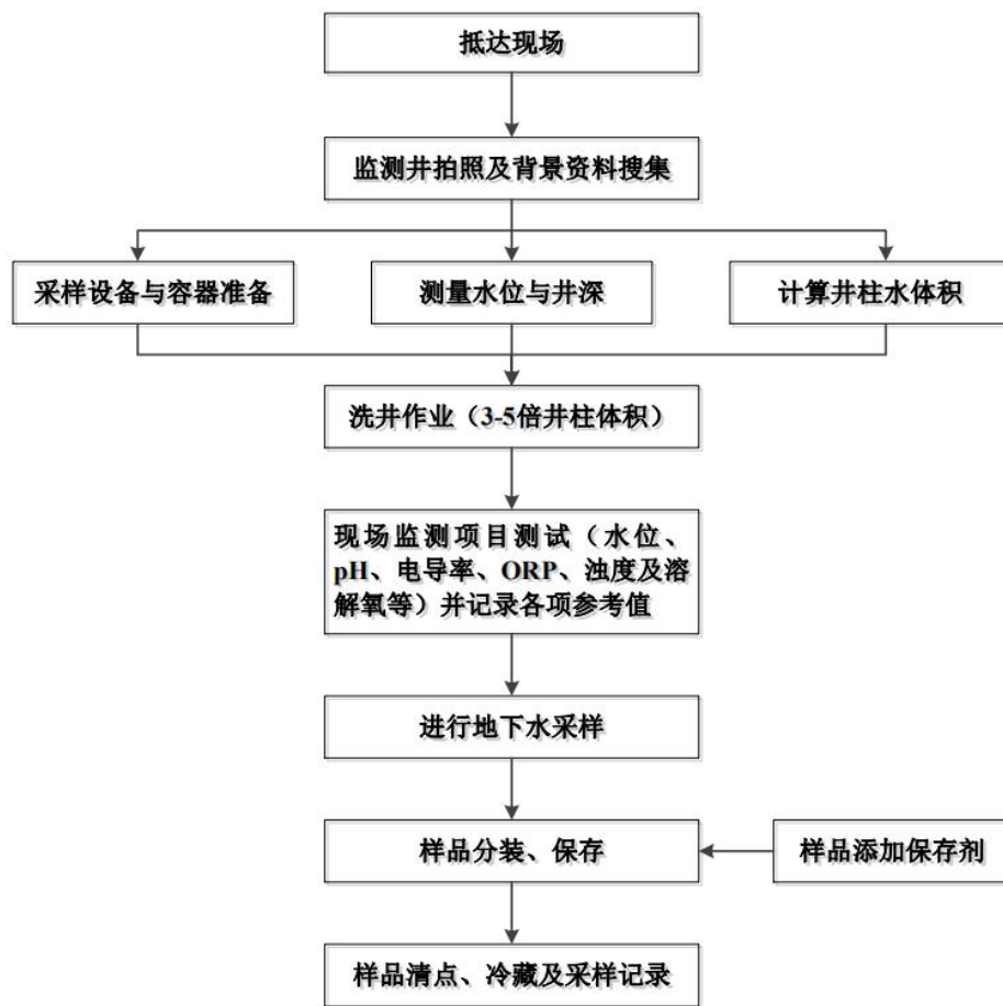
图7.2-1 地下水样品采样流程图
