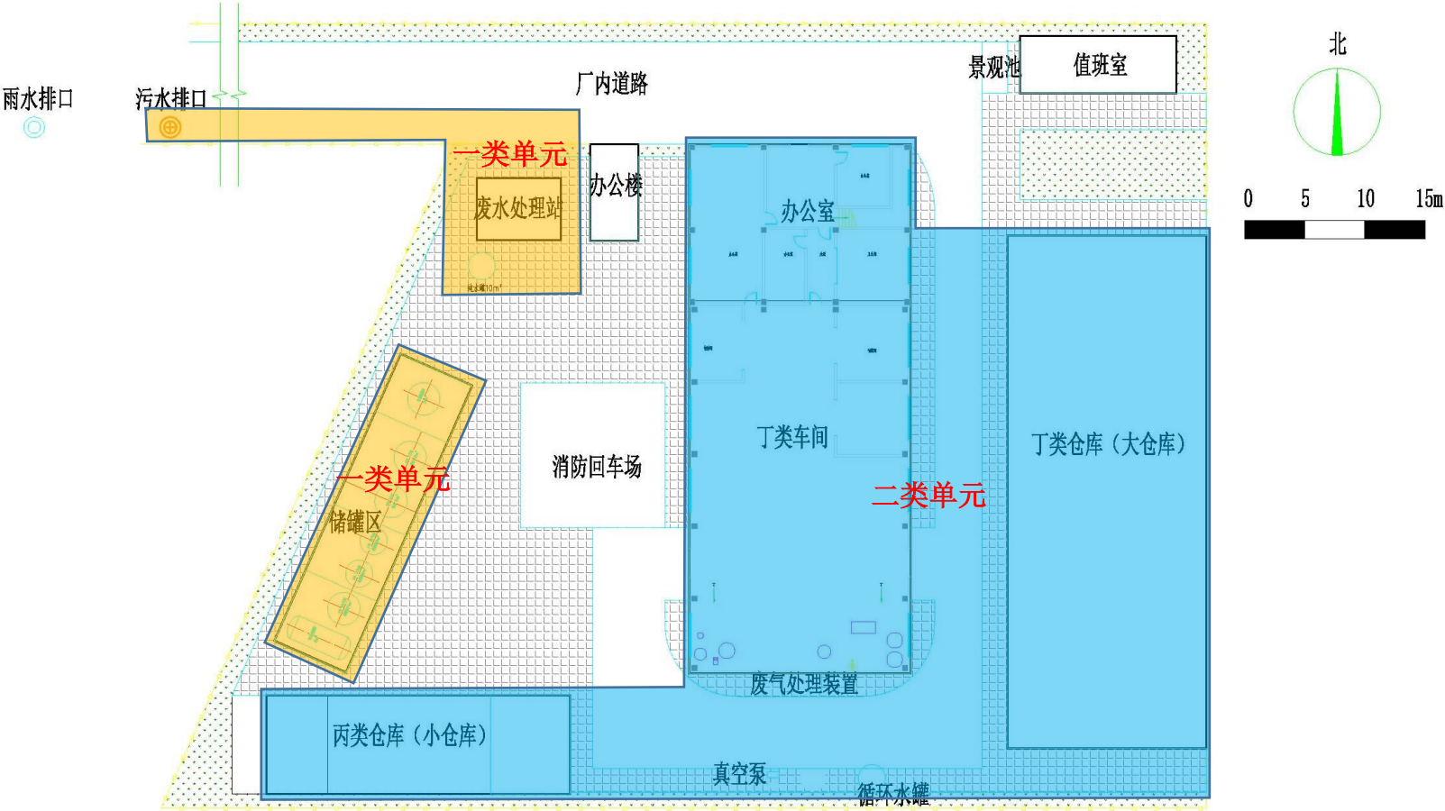
图5.2-1 重点监测单元分区图
