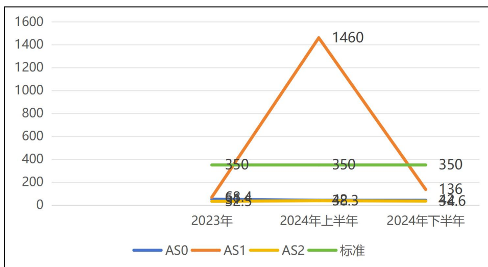
图8.2-5 地下水氯化物变化趋势图 单位：mg/L
