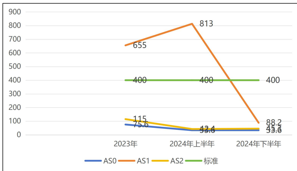
图8.2-8 地下水钠变化趋势图 单位：mg/L
