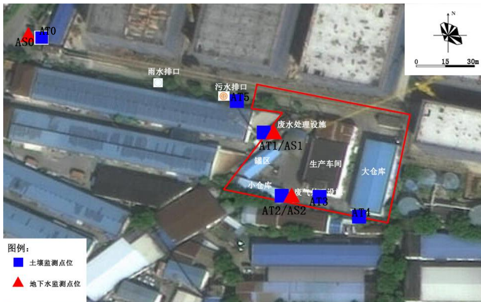
图 6.1-1 项目土壤、地下水监测点位图
