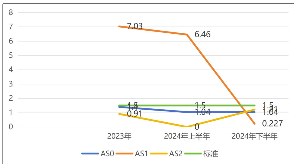
图8.2-6 地下水锰变化趋势图 单位：mg/L
