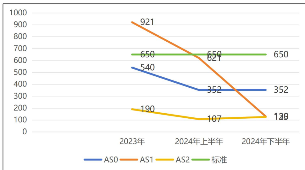
图8.2-3 地下水总硬度变化趋势图 单位：mg/L
