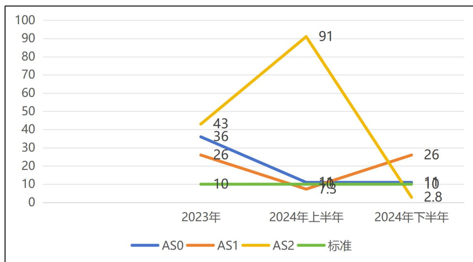
图8.2-1 地下水浊度变化趋势图 单位：NTU
