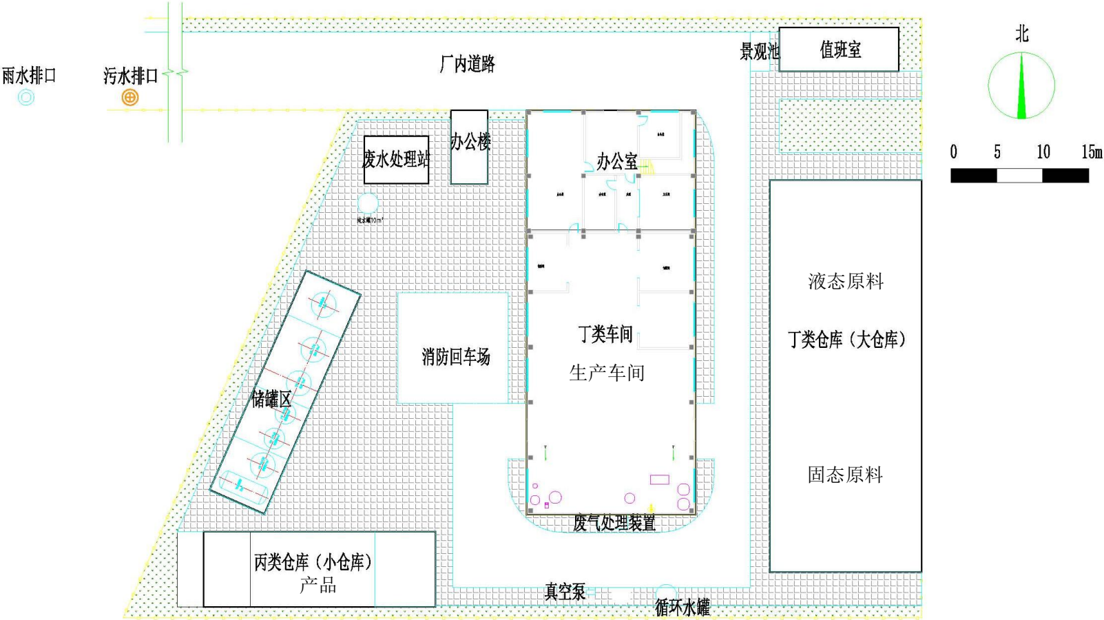
图 4.2-1 项目平面布置图
