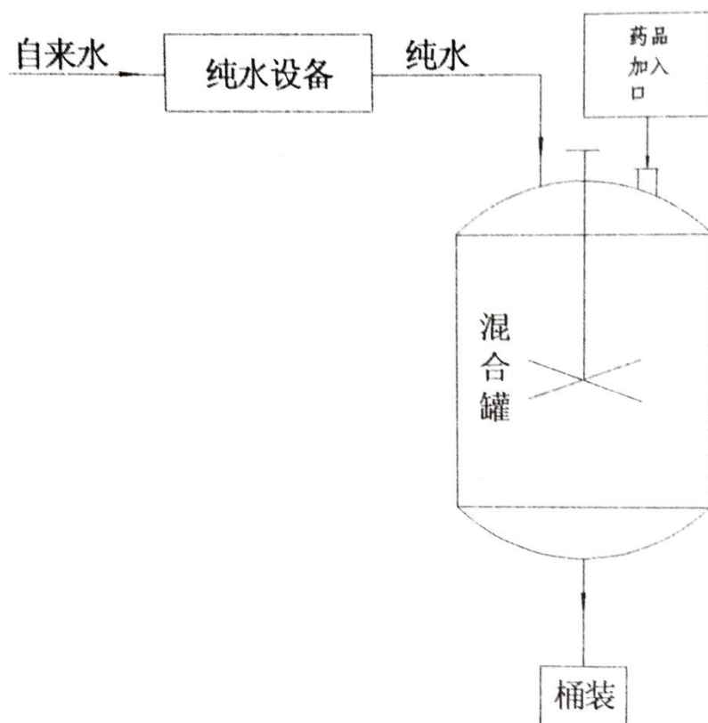
图4.1-1 水处理药剂生产工艺流程图
