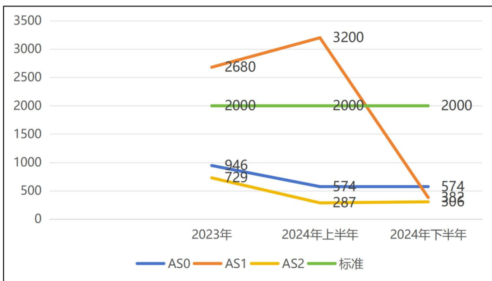
图8.2-2 地下水溶解性总固体变化趋势图 单位：mg/L
