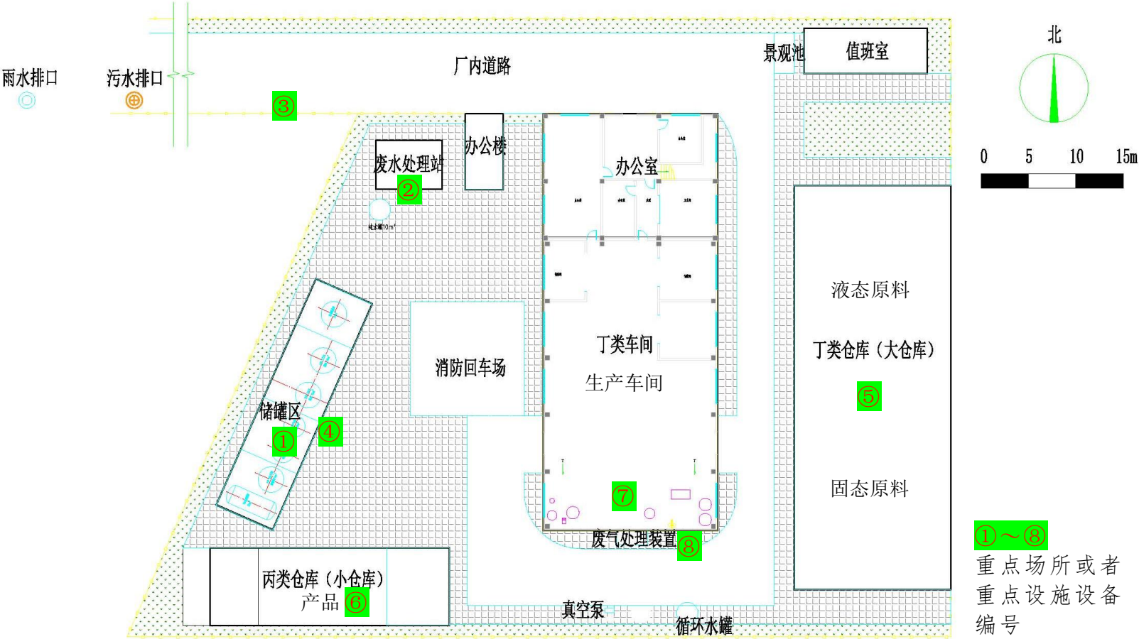
图 4.3-1 重点场所或者重点设施设备分布图
