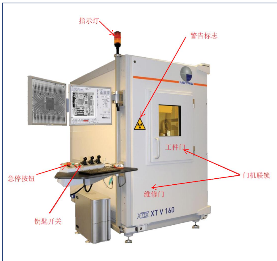
图 10-2 X 射线检测装置辐射安全和防护措施示意图
