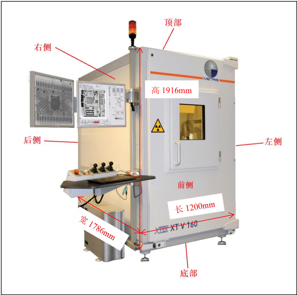
图 9-1 XTV 160 型 X 射线检测装置样式图
