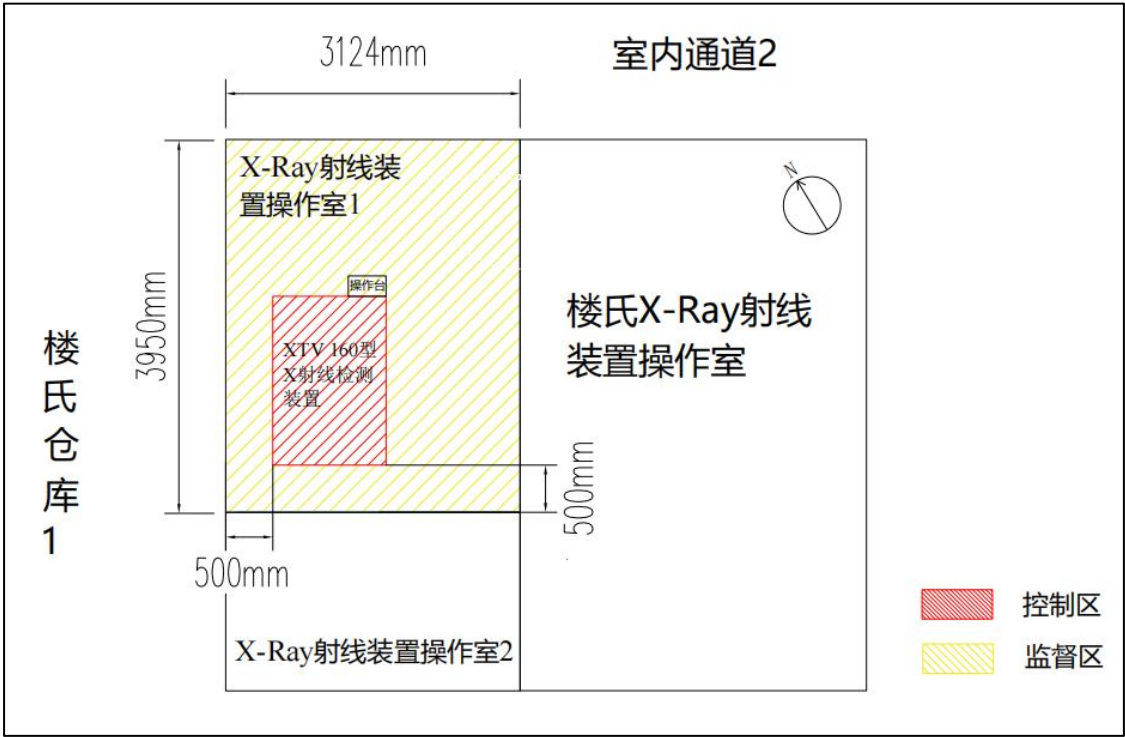
图 10-1 本项目 X 射线检测装置控制分区示意图
