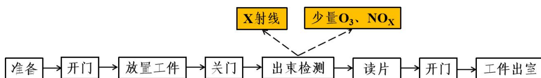
图 9-5 本项目 X 射线检测装置工作流程及产污环节示意图
