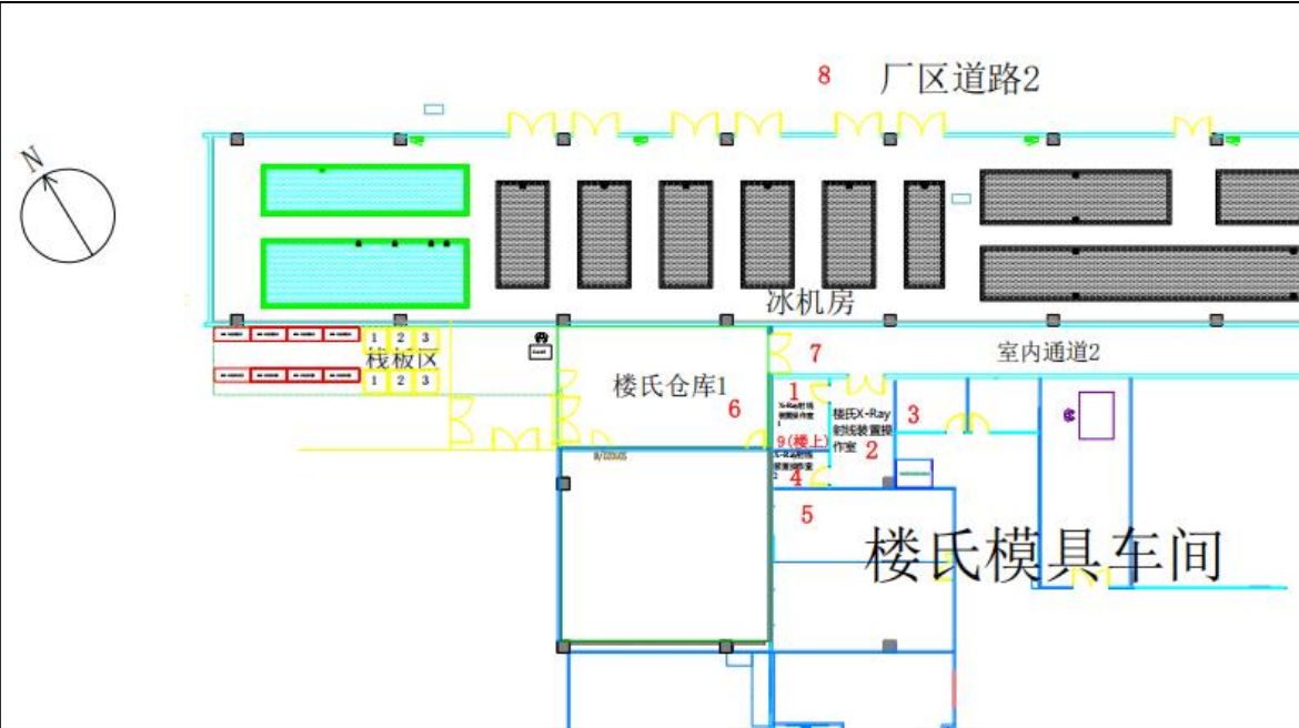
图 8-2 拟建址周围环境γ辐射剂量率监测点位示意图
