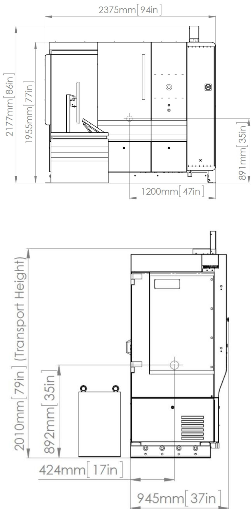
图 9-2 COMET-YXLON FF20 CT 型 X 射线检测系统装置外观尺寸图
