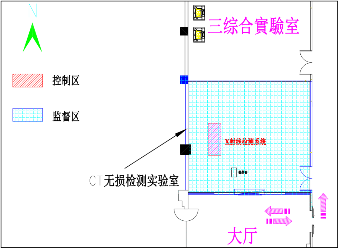
图 10-1 COMET-YXLON FF20 CT 型 X 射线检测系统监督区及控制区示意图
