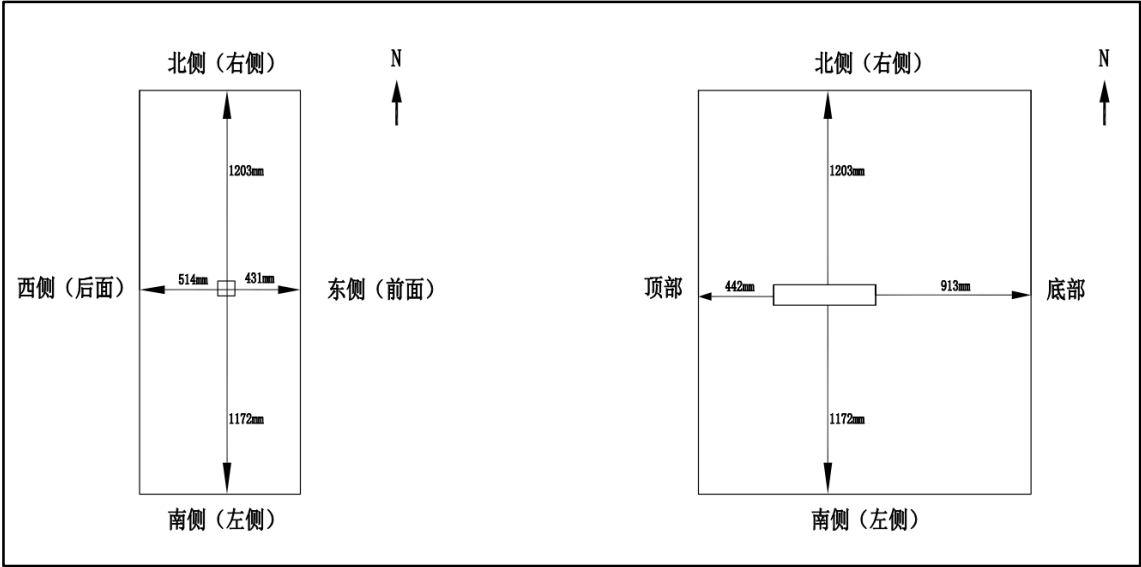
图 11-1 本项目检测装置辐射源点到各侧表面最近距离示意图（单位：mm）
