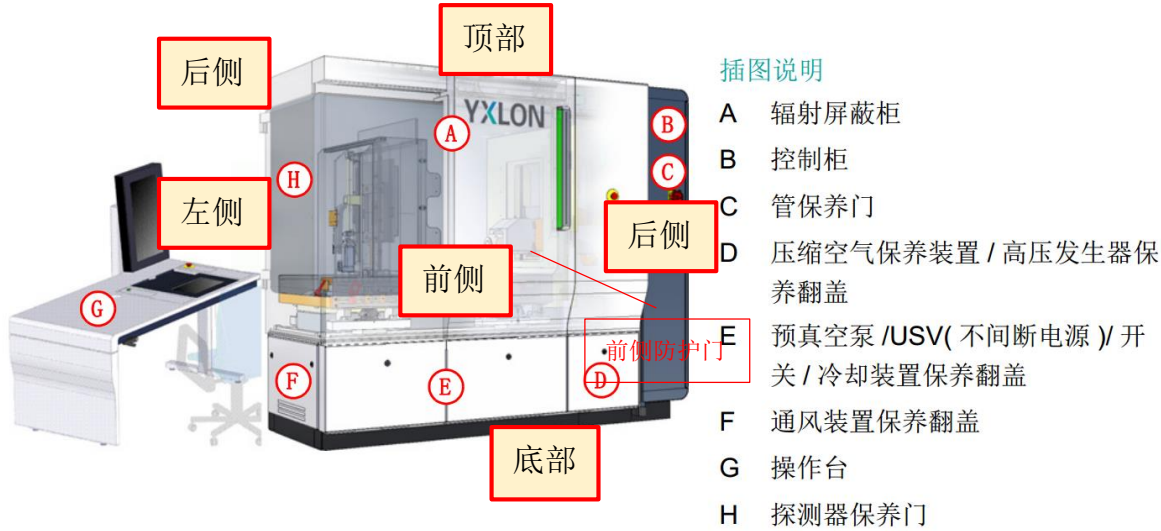
图 9-1 COMET-YXLON FF20 CT 型 X 射线检测系统样式图
