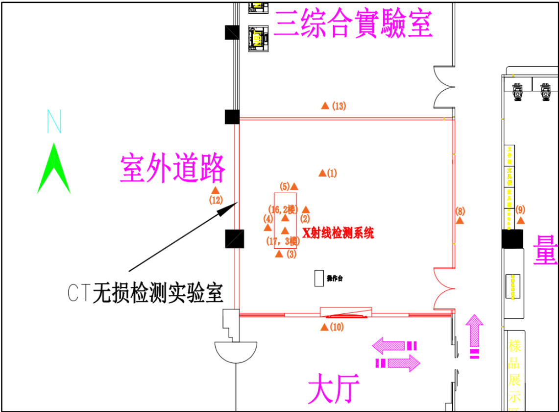
图 11-2 屏蔽计算点示意图
