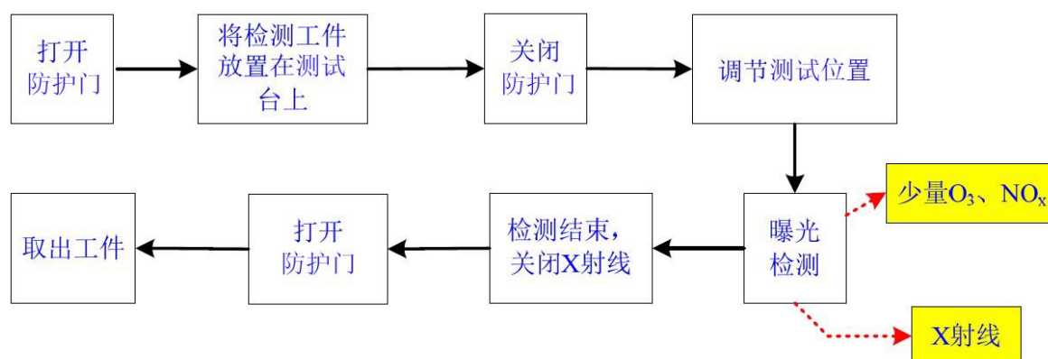
图 9-4 本项目 X 射线检测系统工艺流程及产污环节分析示意图
